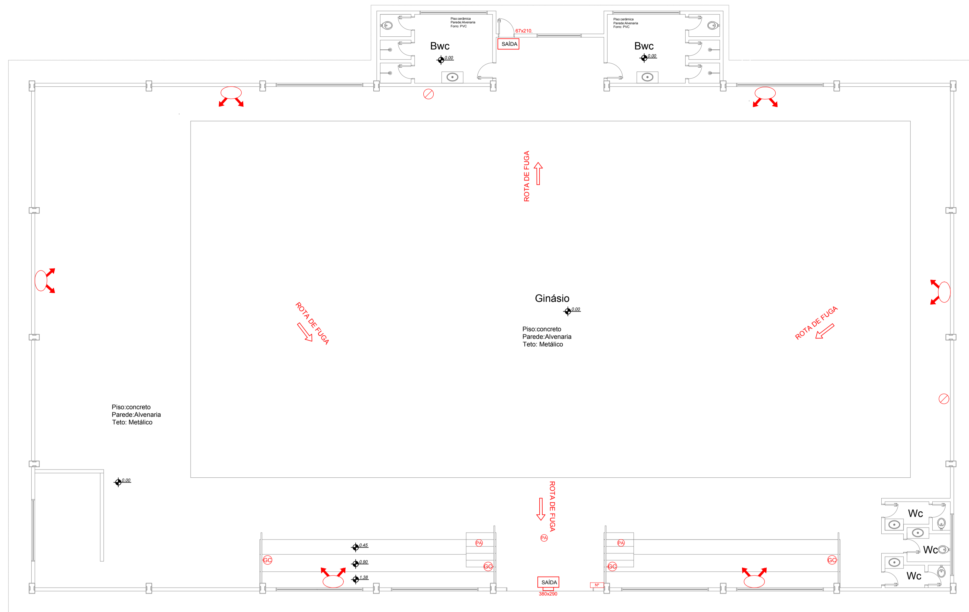
Sistemas de Prevenção Contra Incêndio e plano de emergência - Planta Baixa Escala 1:100
