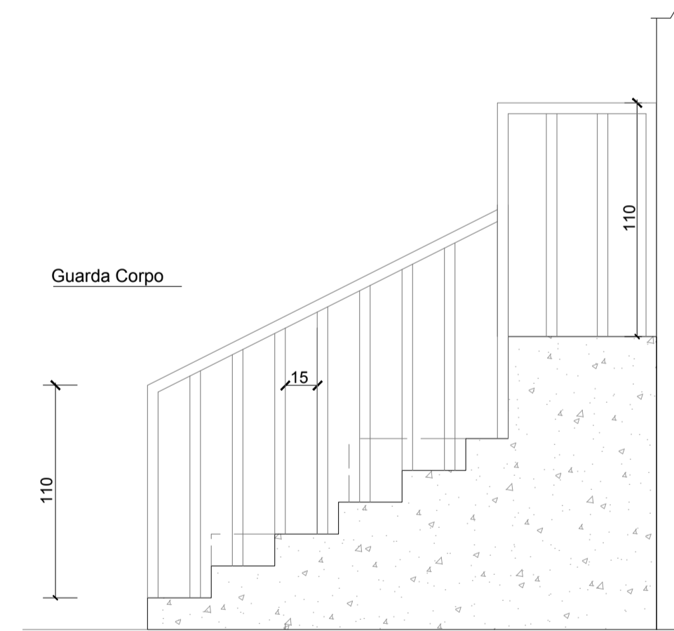
Guarda corpo e Corrimão Sem Escala
