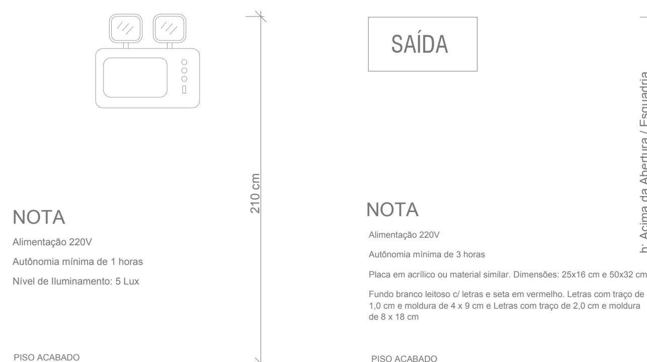
Iluminação de Emergência- Farolete 3000 lumens Sem Escala
