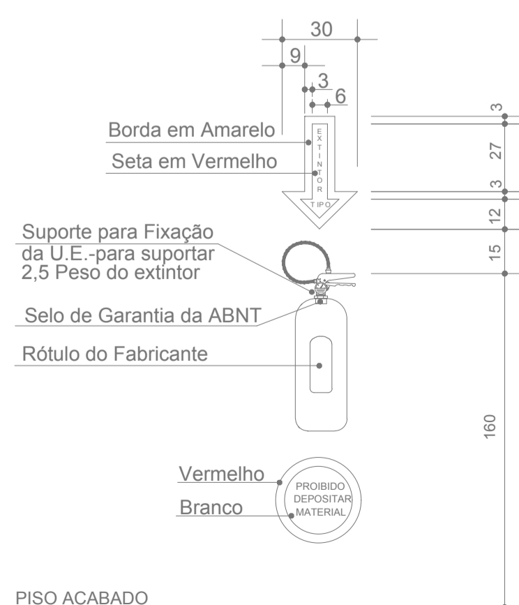
Extintor Sem Escala
