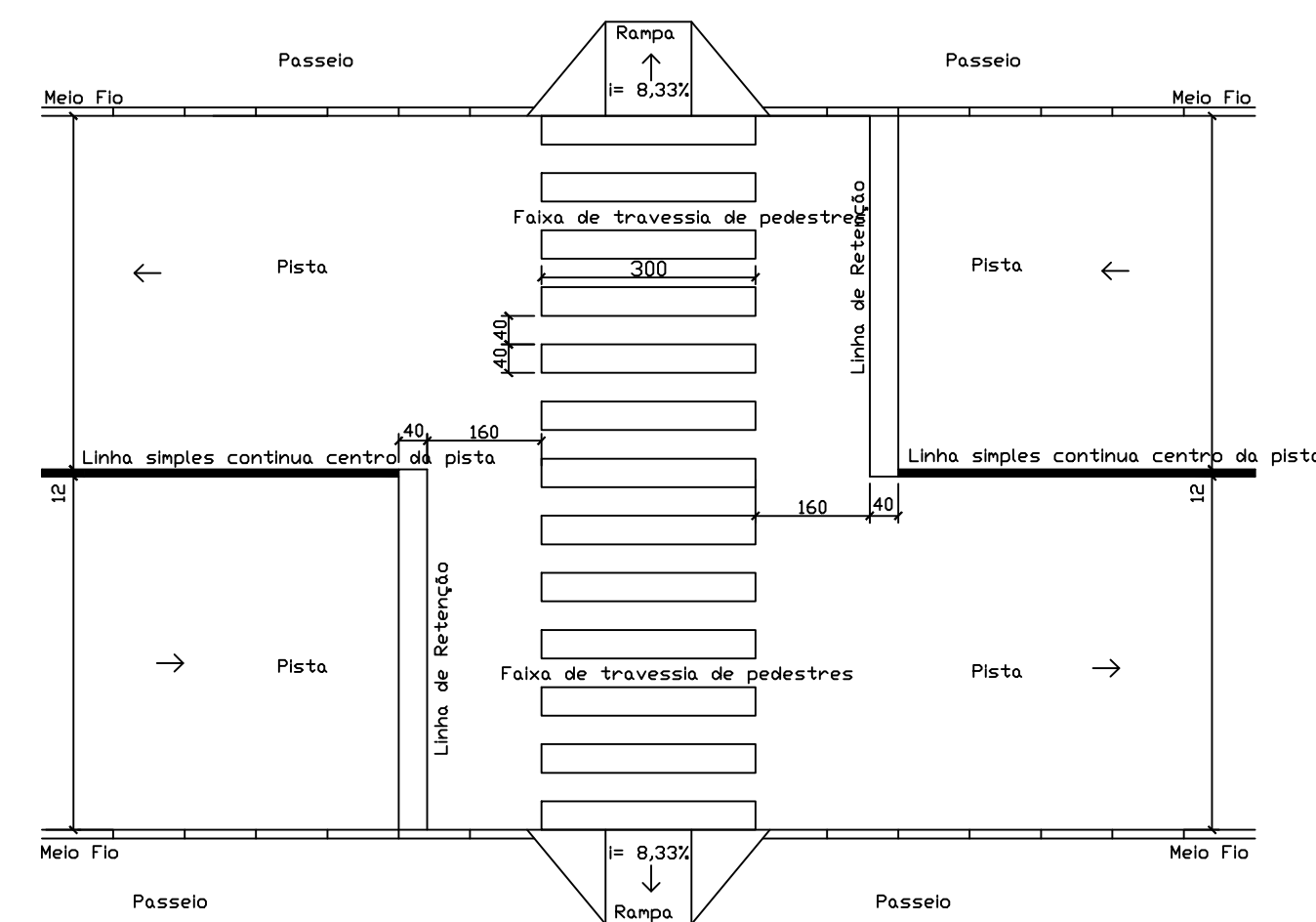
DETALHAMENTO - SINALIZAÇÃO HORIZONTAL
